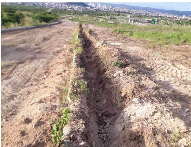
FOTO 02: RUA PROJETADA R-1 (AO LADO DA QUADRA C, ESCAVAÇÃO PARA REDE DE ESGOTO).
